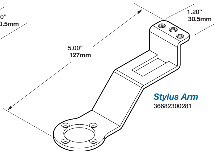
Stylus Arm
