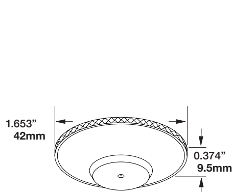
CL Nut
