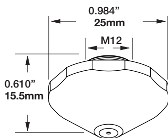
Nozzle EAA
